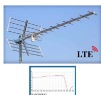
DL13/LTE ANTENNA UHF 13 ELEMENTI 21-60 470-790 MHZ 114 CM 8-13 DB
